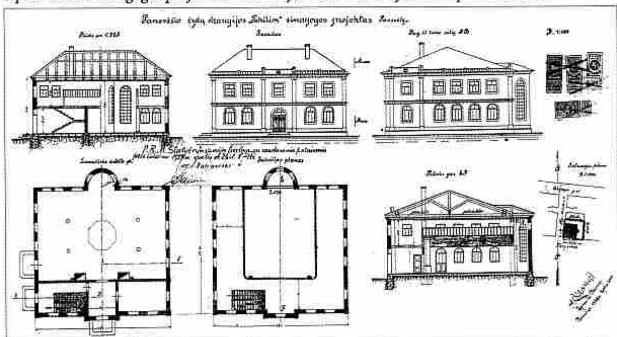
5 pav. Tehilim sinagogos projektas. Panevėžys. 1929. LCVA, f. 1622, ap. 4, b. 39, l. 8
