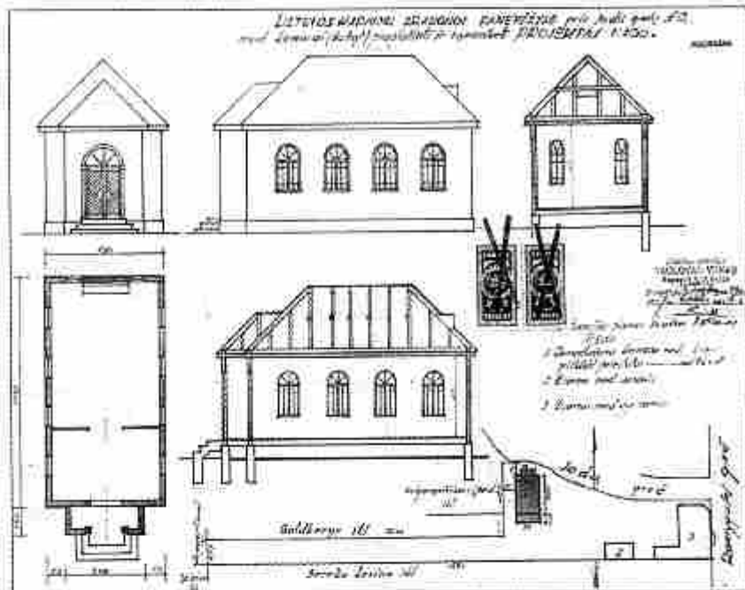
9 pav. Karaimų kenesos projektas. Panevėžys. LCVA, f. 1622, ap. 4, b. 713, l. 60
